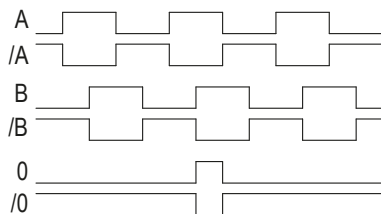
Abb. 4: Impulsbild
