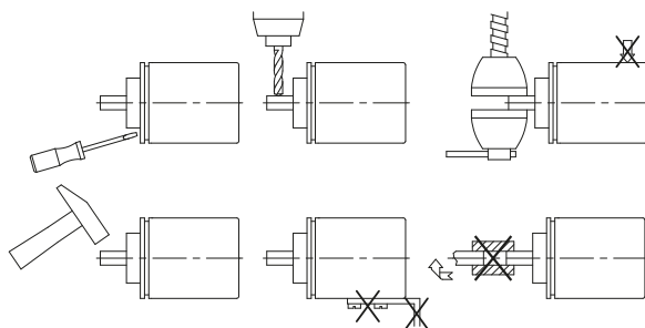
Abb. 1: Montagehinweise
