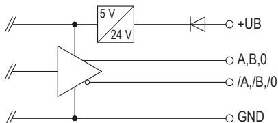
Abb. 3: Ausgangsschaltung LD24
