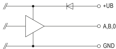
Abb. 2: Ausgangsschaltung PP
